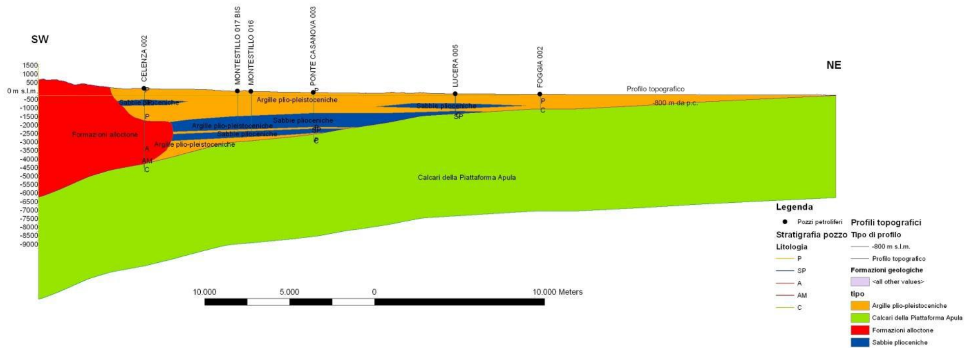
Fig. B.15 – Sezione geologica FF'.
