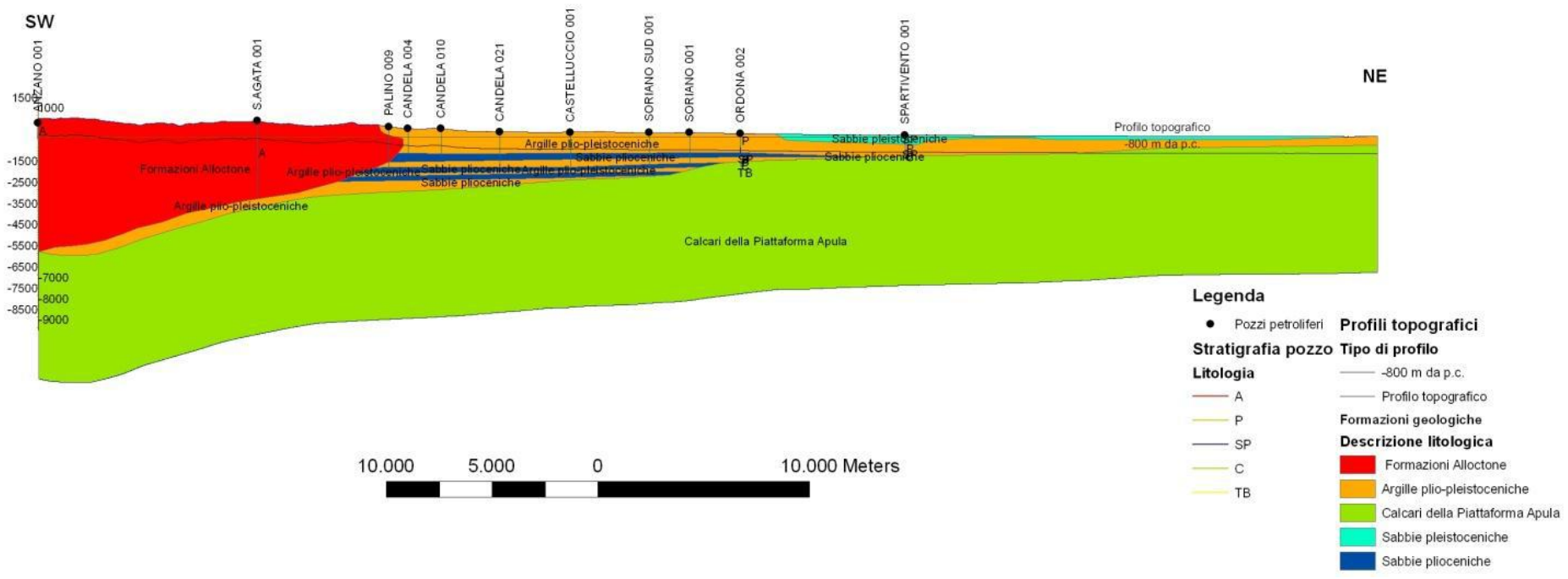
Fig. B.21 – Sezione geologica NN'.
