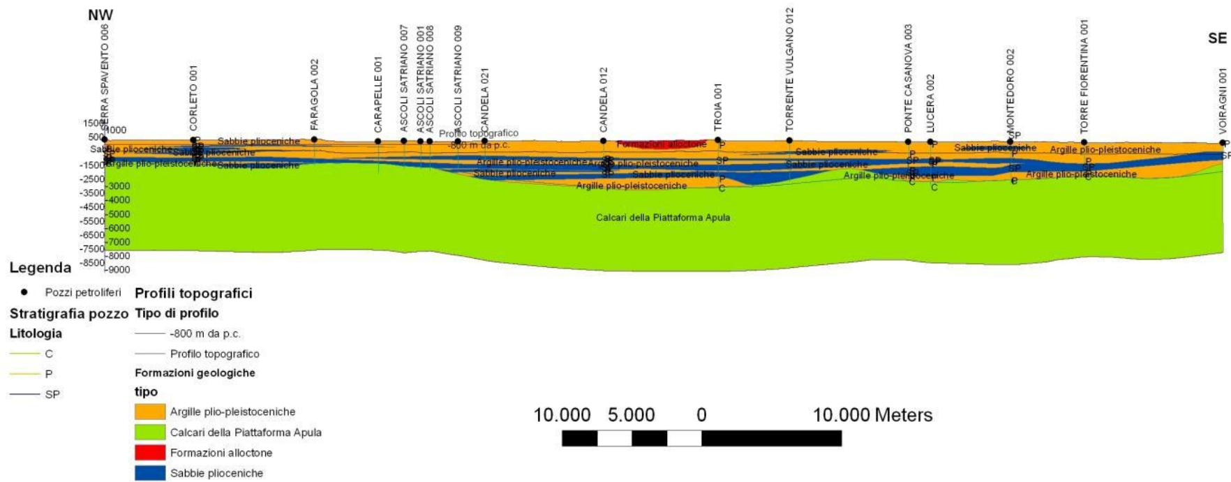
Fig. B.31 – Sezione geologica WW'.
