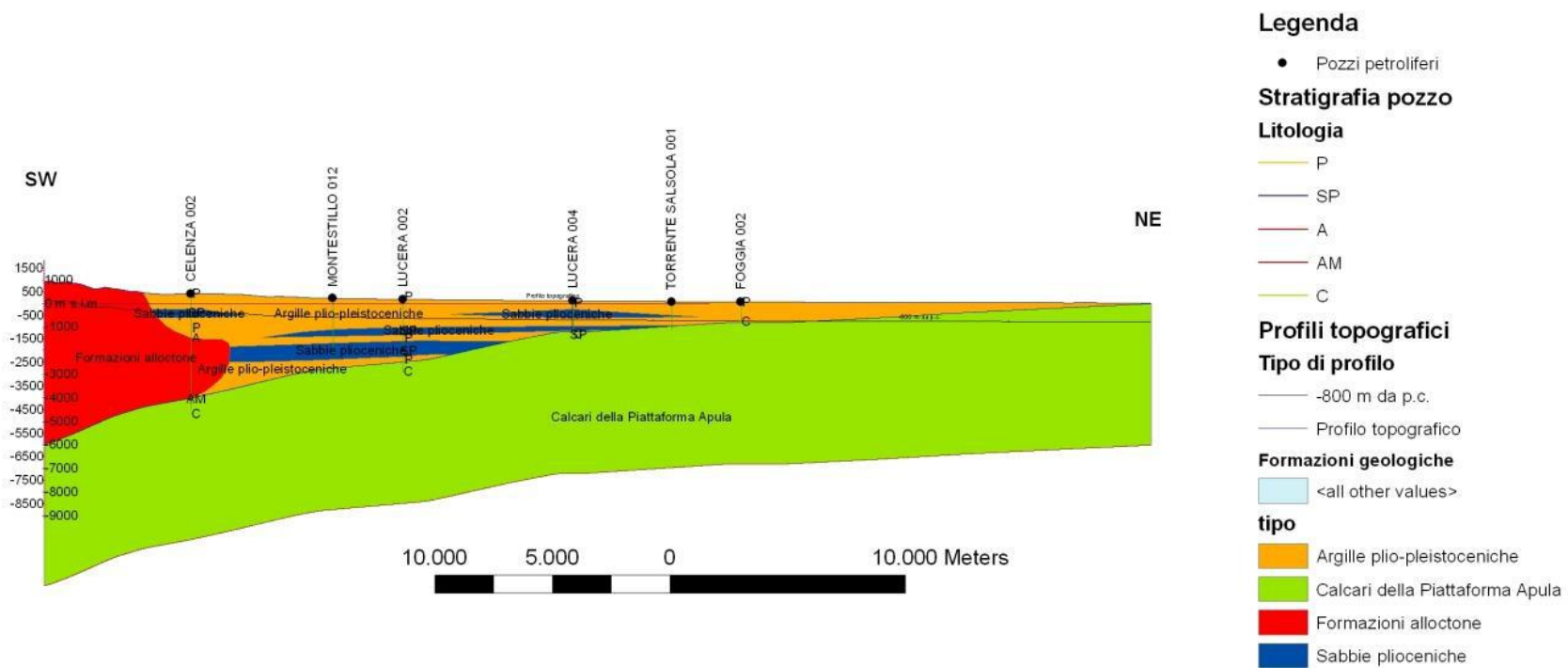
Fig. B.11 – Sezione geologica EE'.
