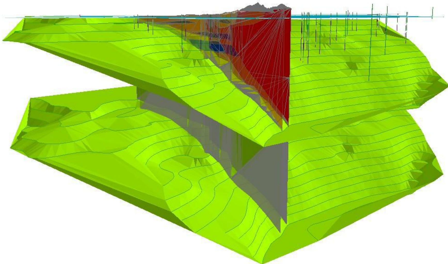
Fig. B.5 – Modello geologico 3D per le sezioni BB' e CC'.
