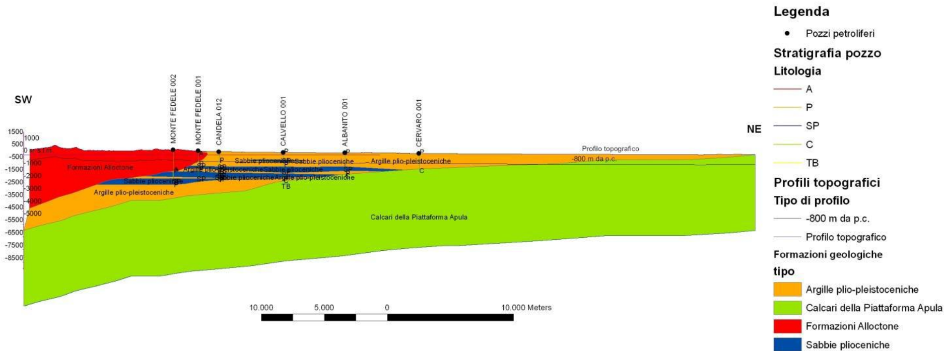
Fig. B.20 – Sezione geologica MM'.
