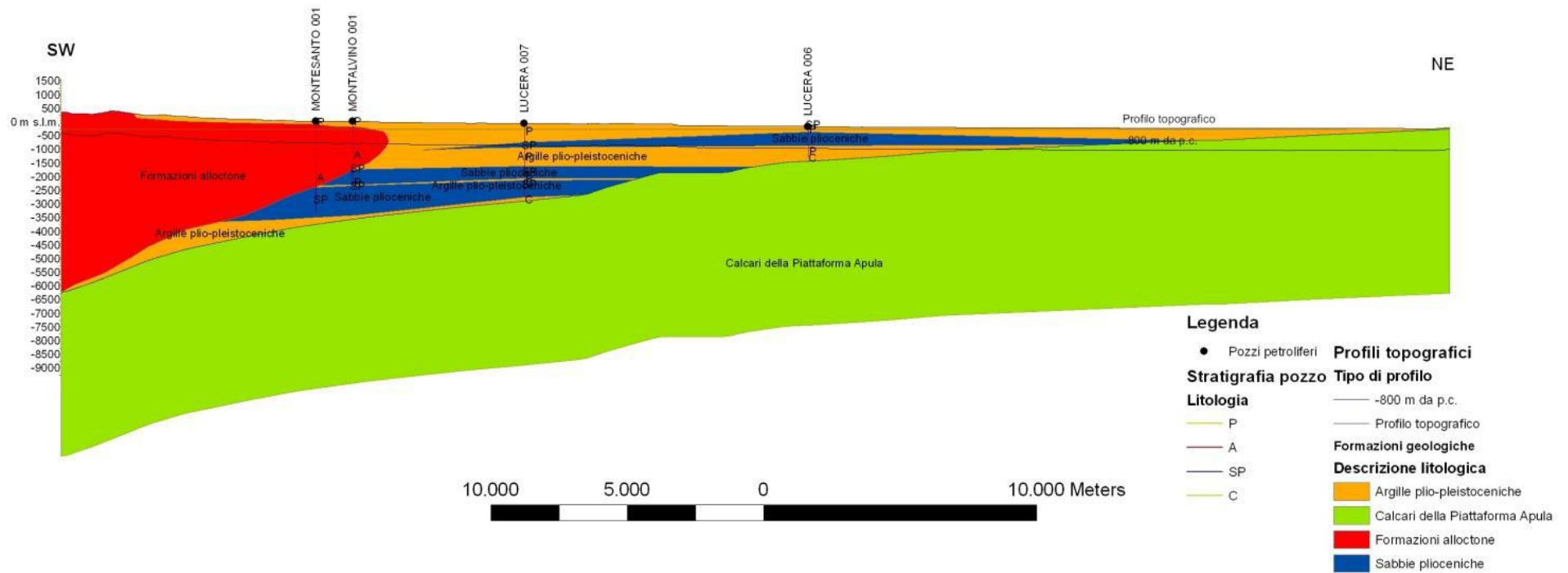
Fig. B.17 – Sezione geologica HH'.
