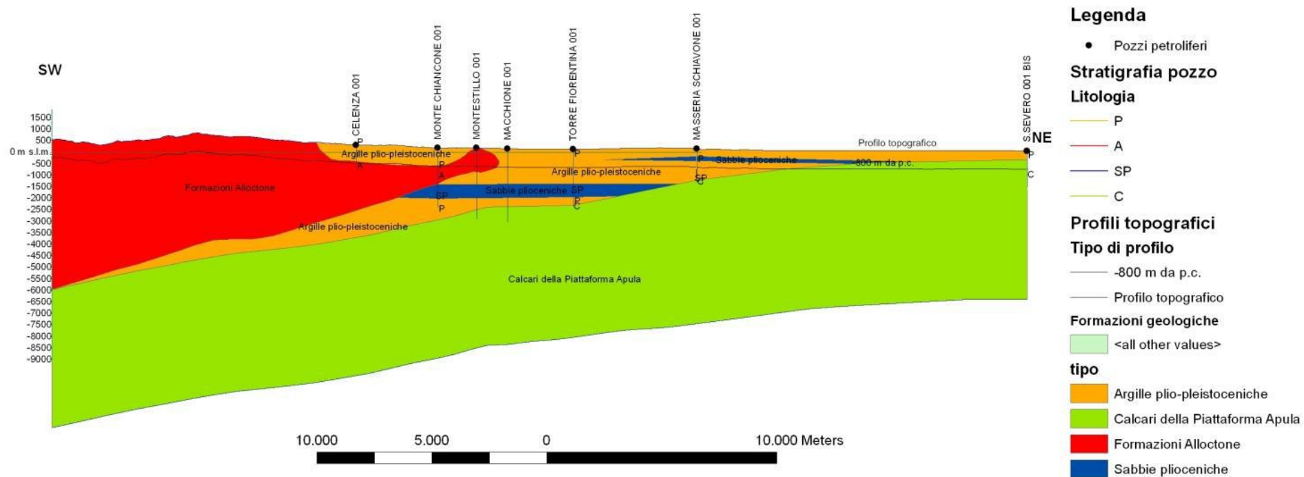
Fig. B.2 – Sezione geologica BB'.
