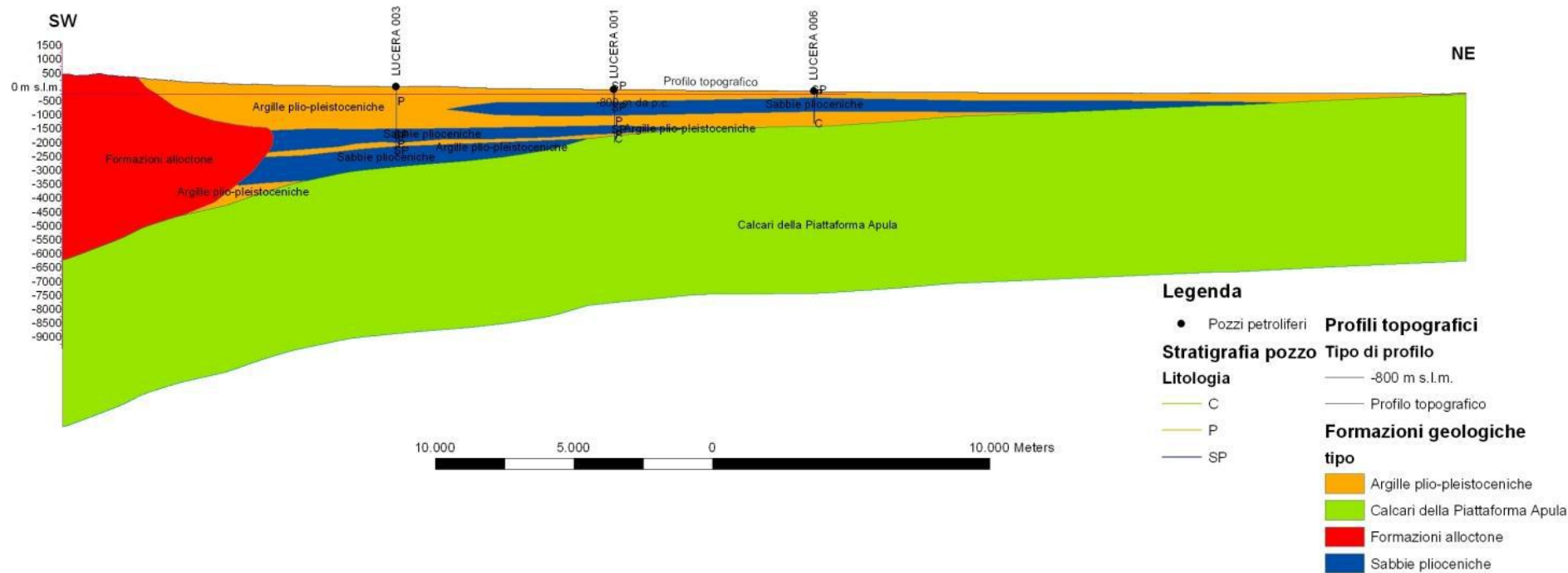
Fig. B.16 – Sezione geologica GG'.
