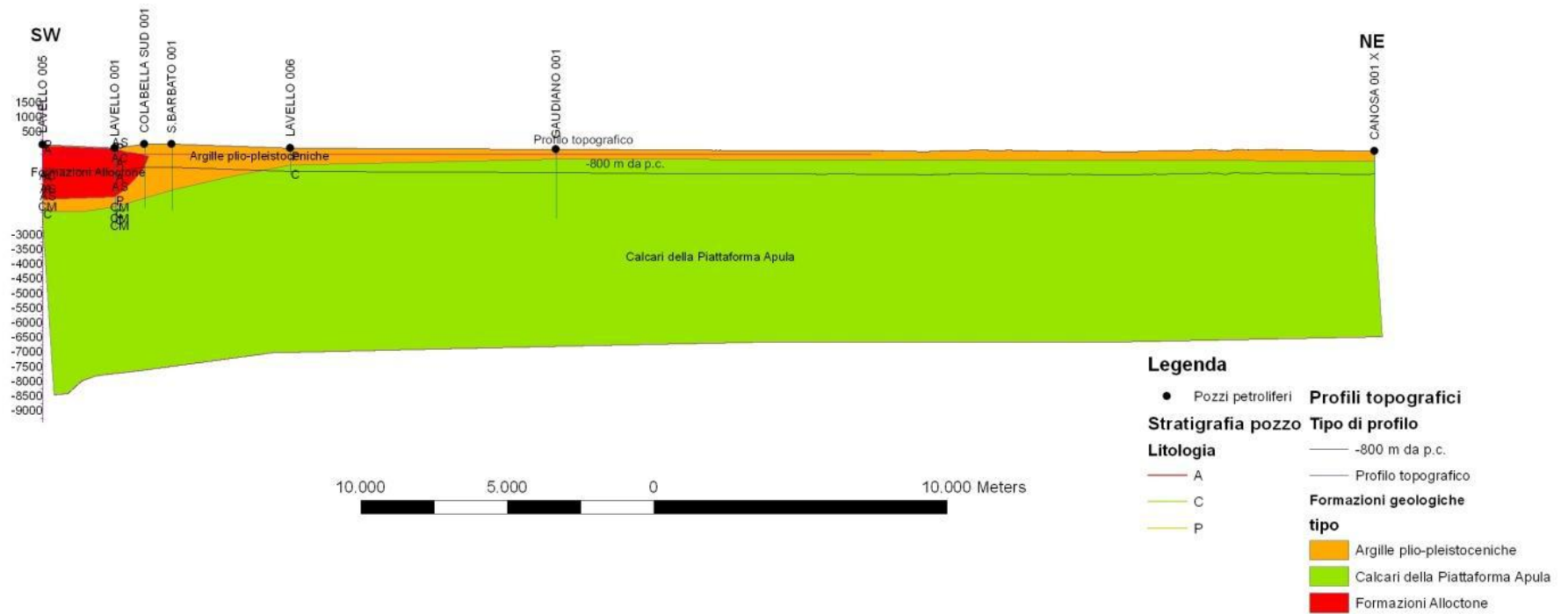
Fig. B.26 – Sezione geologica SS'.
