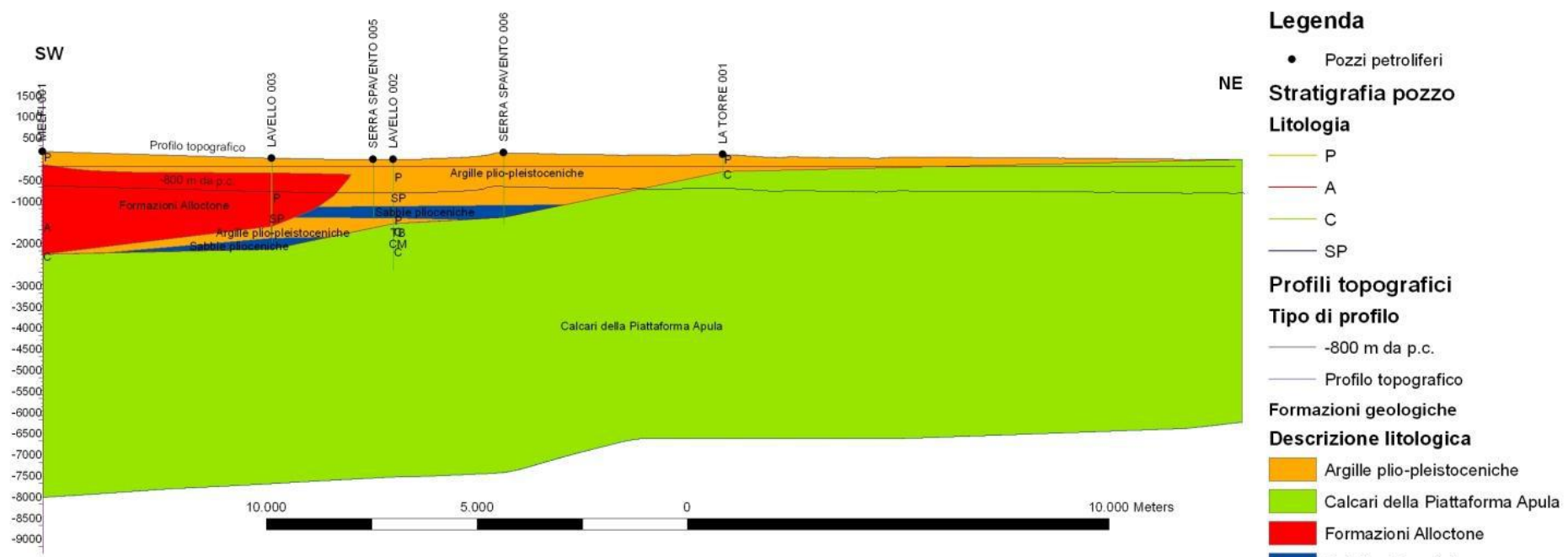
Fig. B.24 – Sezione geologica QQ'.
