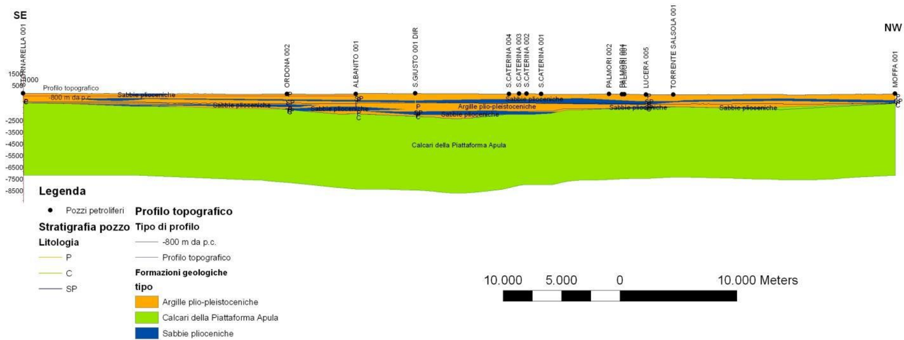
Fig. B.32 – Sezione geologica JJ'.
