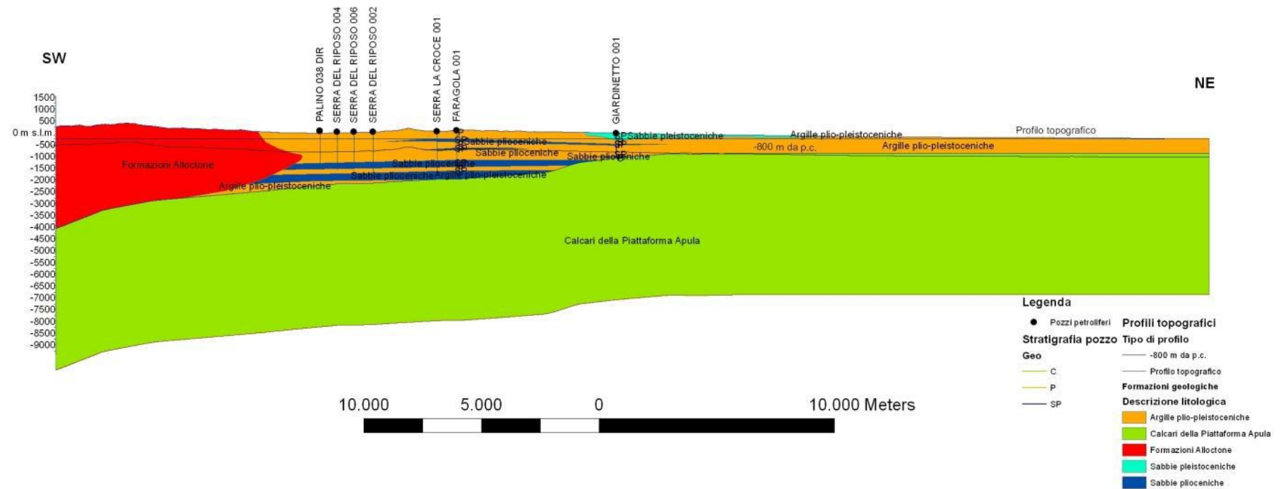
Fig. B.22 – Sezione geologica OO'.
