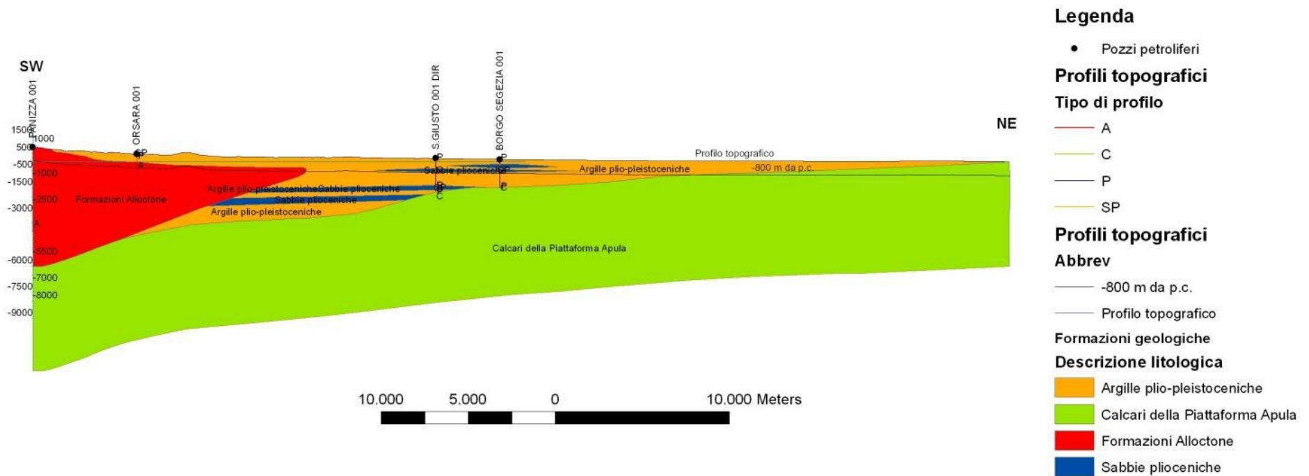
Fig. B.19 – Sezione geologica LL'.
