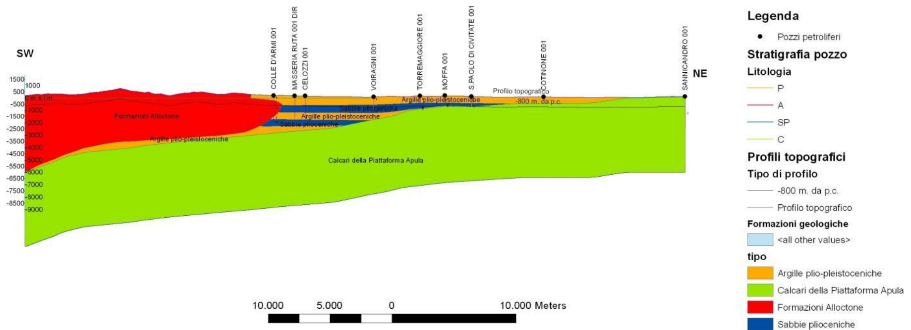
Fig. B.1 – Sezione geologica AA'.
