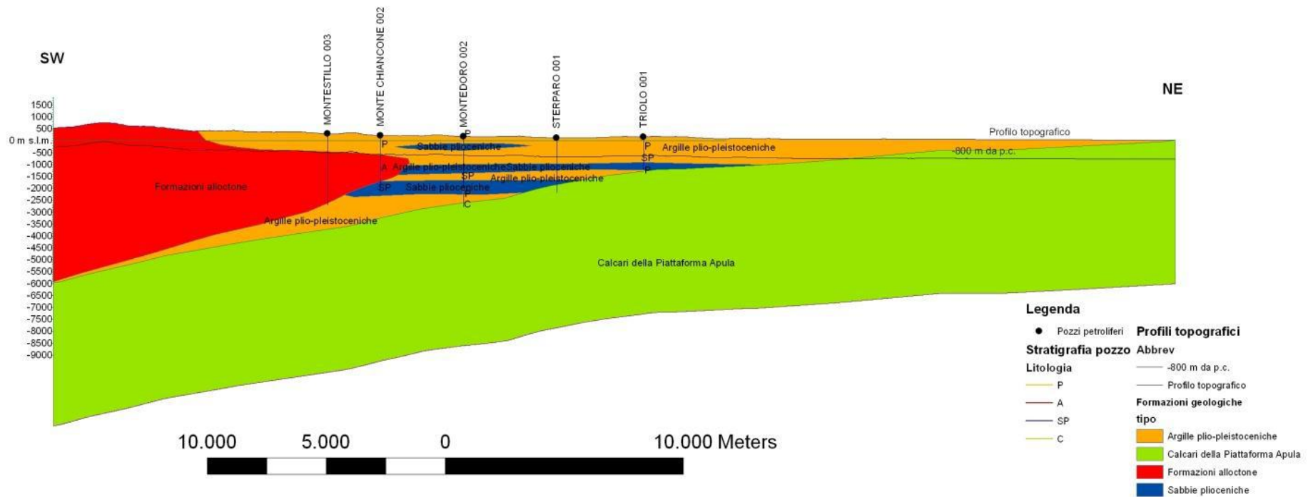
Fig. B.4 – Sezione geologica CC'.
