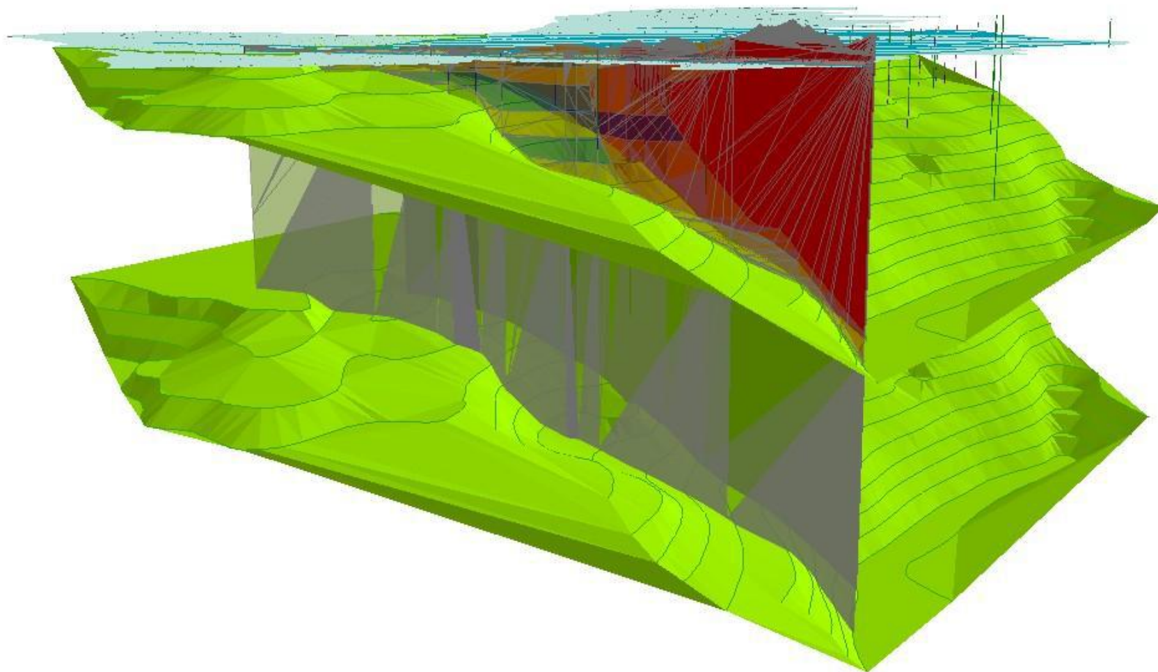
Fig. B.3 – Modello geologico 3D per le sezioni geologiche AA' e BB' (la sezione AA' è in trasparenza).
