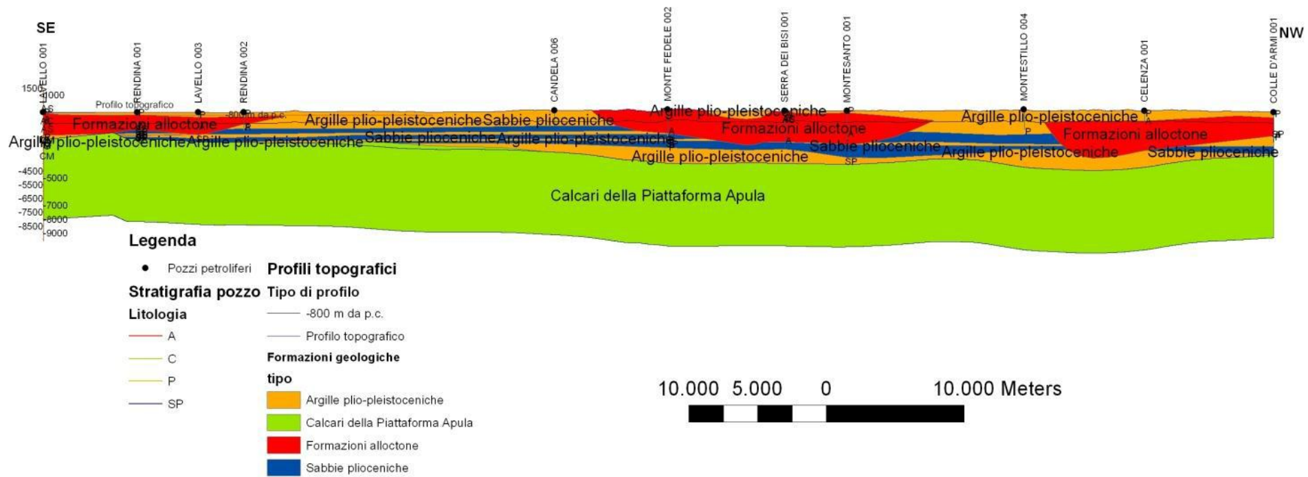
Fig. B.29 – Sezione geologica ZZ'.
