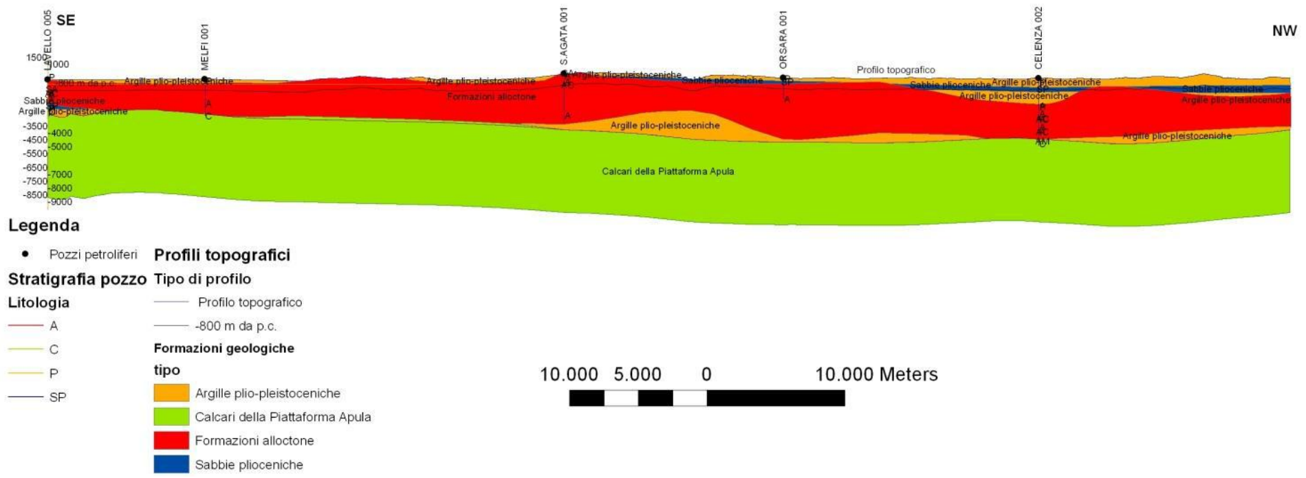
Fig. B.28 – Sezione geologica VV’.
