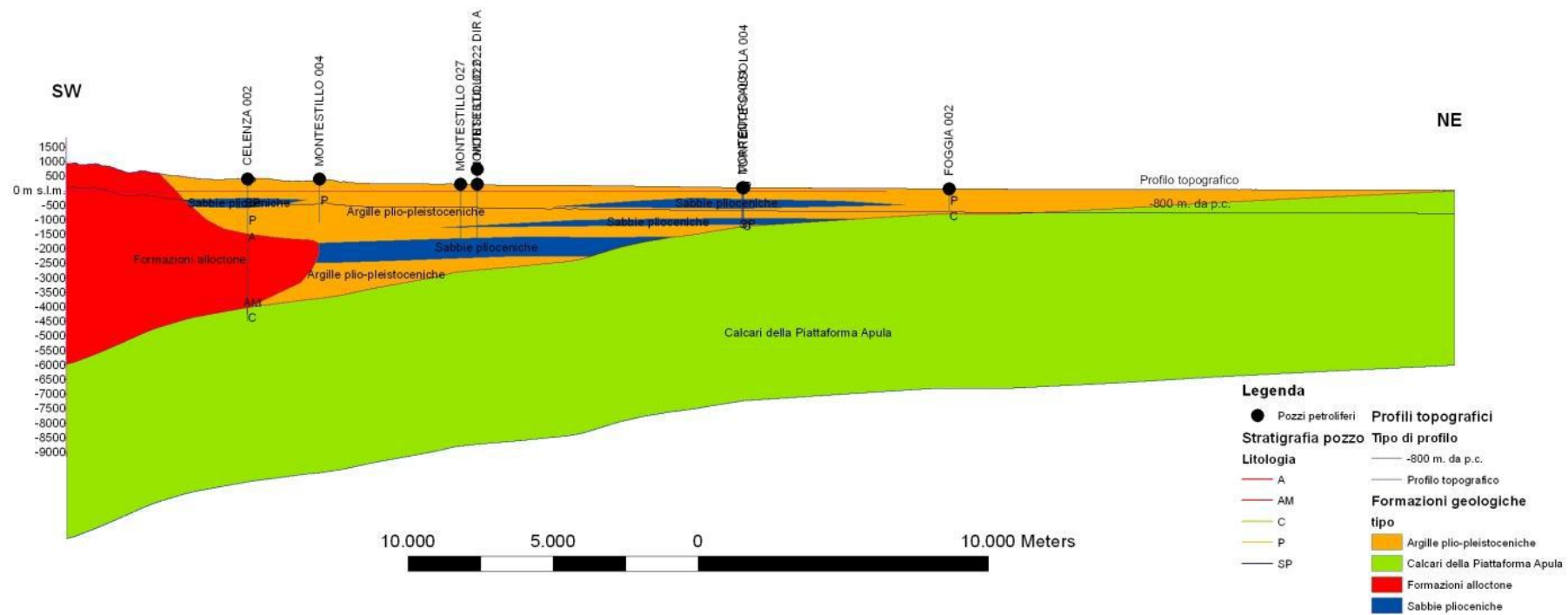
Fig. B.8 – Sezione geologica DD'.
