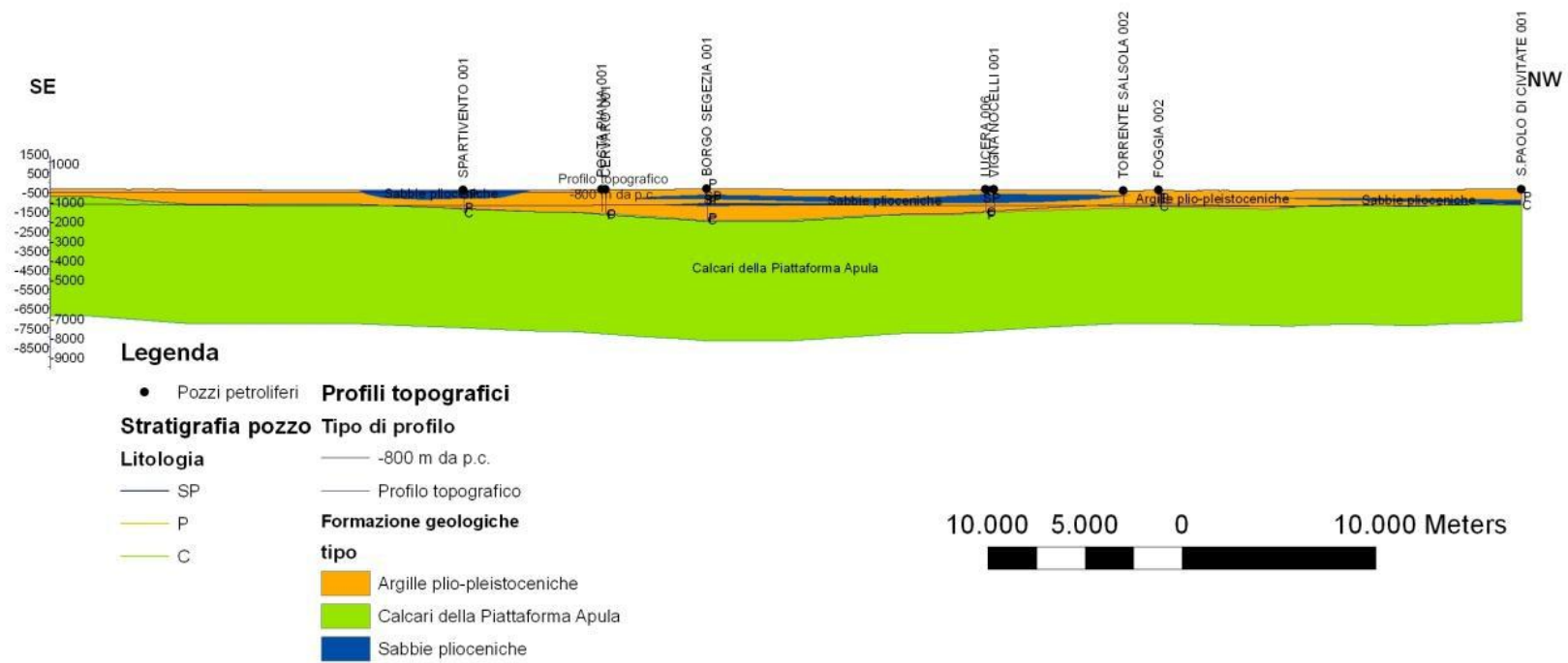
Fig. B.33 – Sezione geologica YY'.
