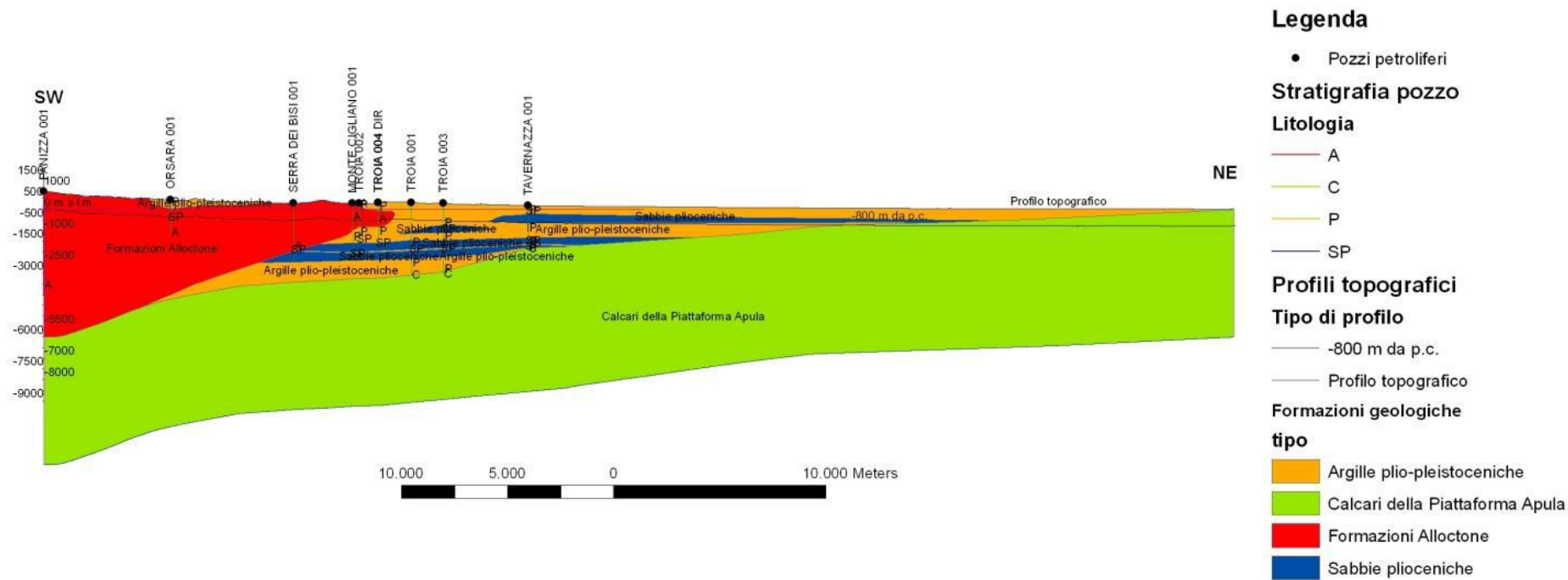
Fig. B.18 – Sezione geologica II'.
