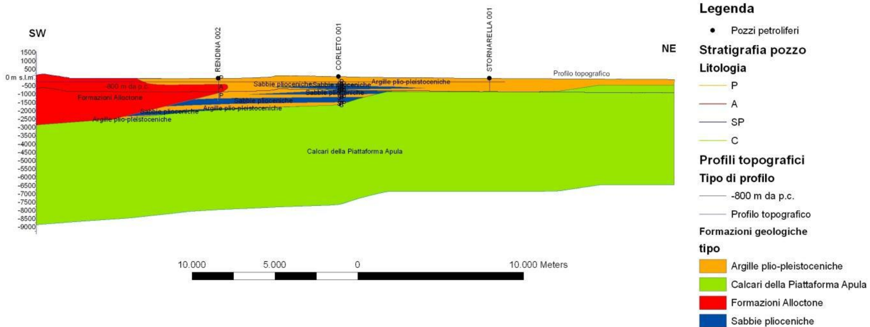
Fig. B.23 – Sezione geologica PP'.
