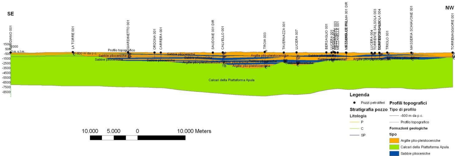
Fig. B.32 – Sezione geologica UU'.
