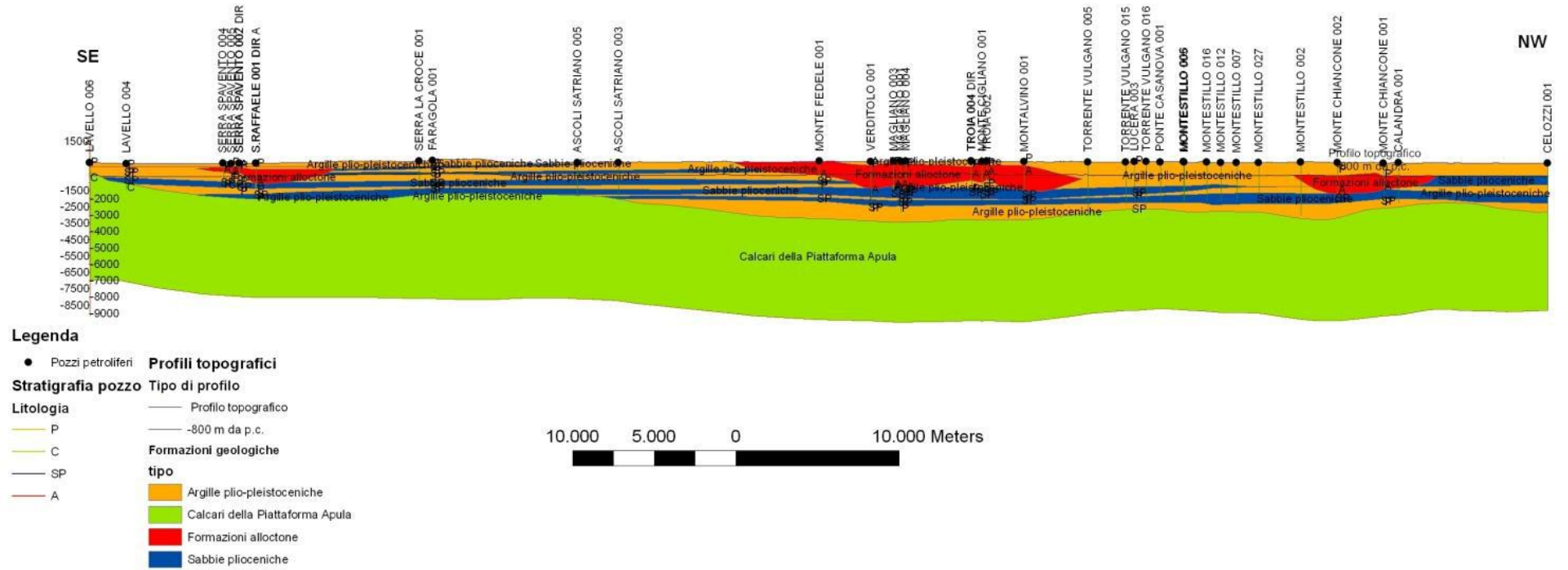
Fig. B.30 – Sezione geologica XX’.
