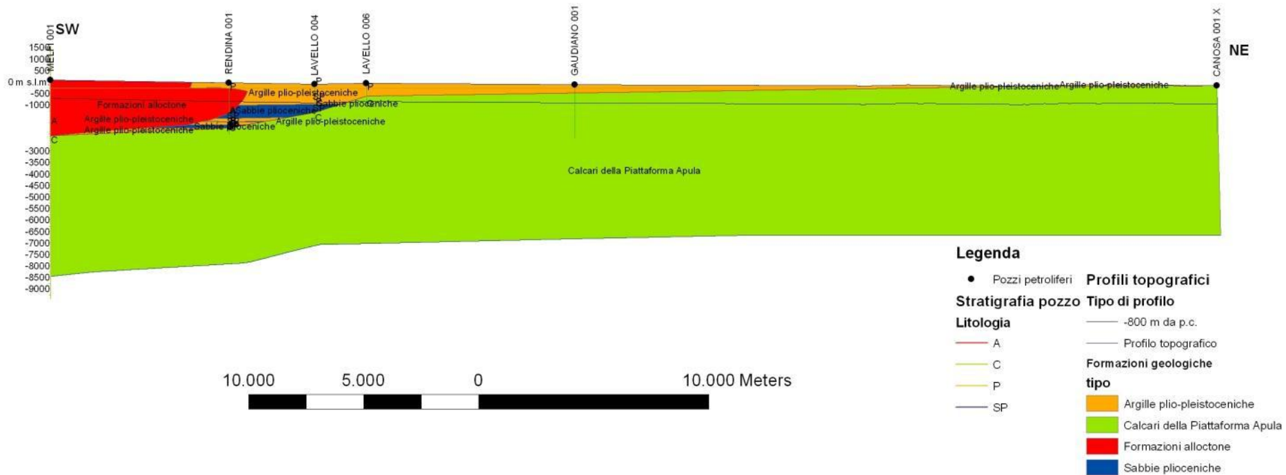
Fig. B.25 – Sezione geologica RR'.
